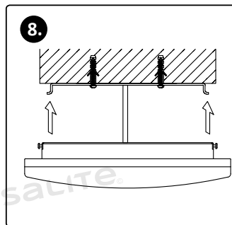
Instalati lampa pe perete!
