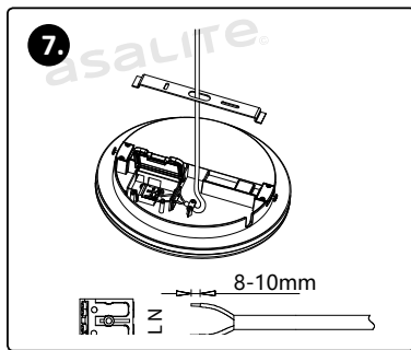
Nyissa ki a csatlakozó dobozt. Kösse be a vezetékeket. Zárja vissza a csatlakozó dobozt. Rögzítse a csavarokat!
