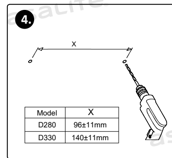
Praticare dei fori in base alla posizione di installazione!
