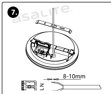
Otvorite razvodnu kutiju. Spojite žice. Pokrijte razvodnu kutiju. Zaključajte vijke!
