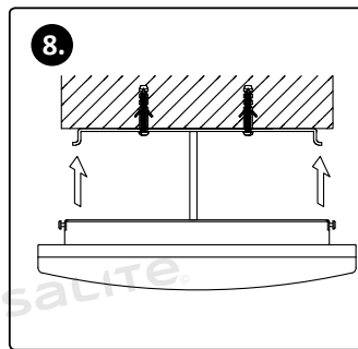
Rögzítse a lámpát a falra!
