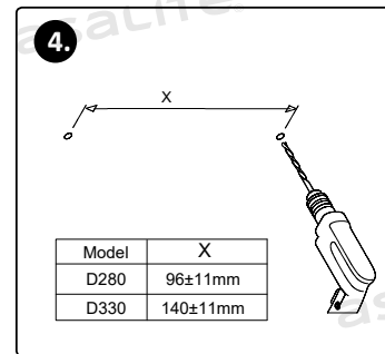
Gauriti gaurile in functie de pozitia de instalare!
