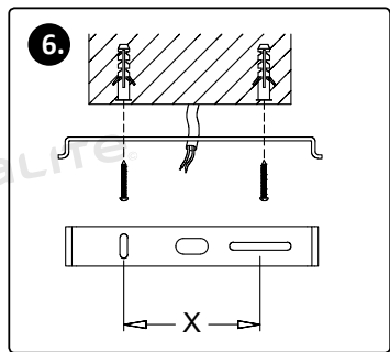
Rögzítse a csavarokat!
