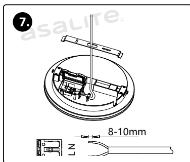
Öffnen Sie die Anschlussdose. Schließen Sie die Drähte an. Decken Sie die Anschlussdose ab. Verriegeln Sie die Schrauben!
