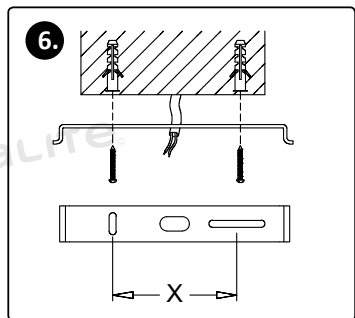
Ugradite vijke!
