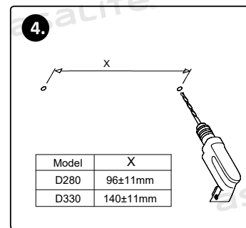
Izvrtaite luknje glede na položaj namestitve!
